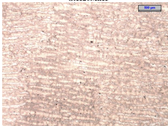
GX120Mn13
