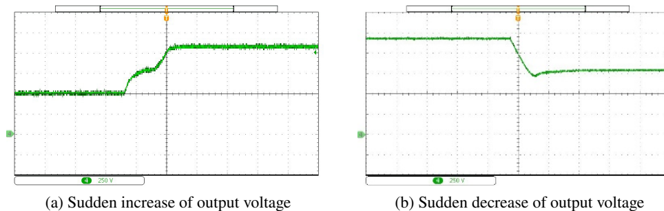
Fig. 16. Output voltage mutation
