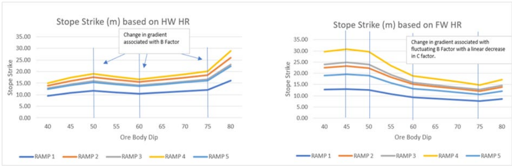
Fig. 20. Slope design parameters for ramps
