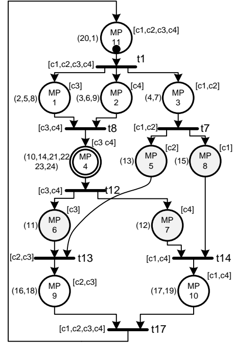
Fig. 3. Petri macronet.
