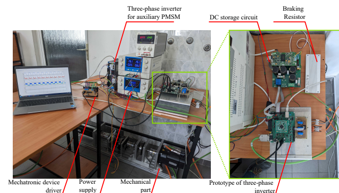
Fig. 9. Laboratory stand
