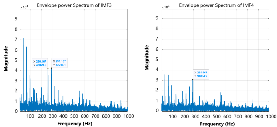
Fig. 27. Envelope spectrum of IMF3-IMF4
