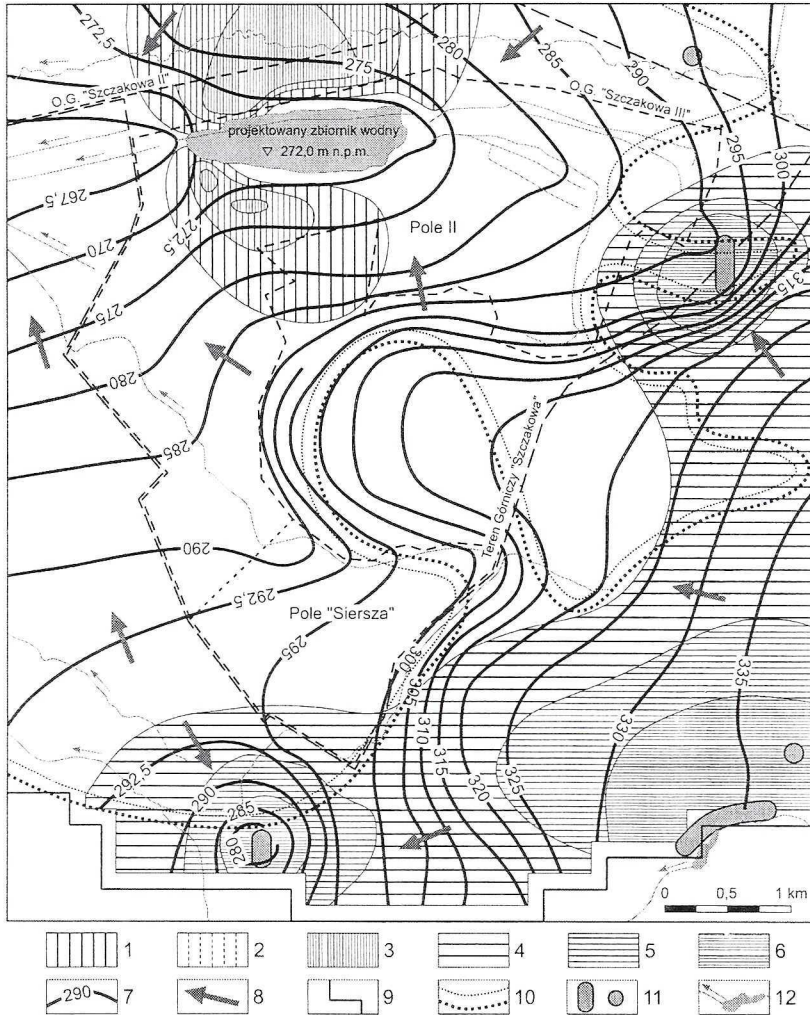
Rys. 3. Mapa hydroizohips czwartorzędowo-triasowego piętra wodonośnego w rejonie obszaru górniczego Szczakowa III – wariant 3
