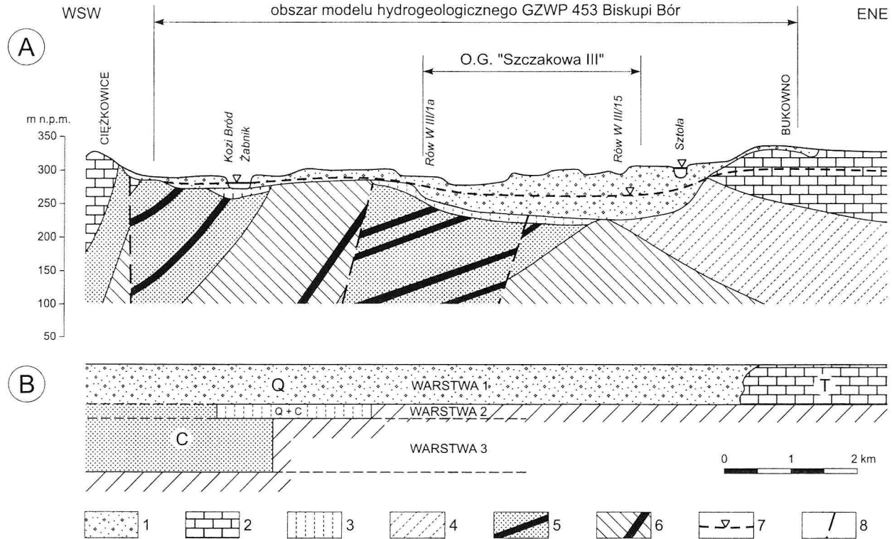
Rys. 2. Schematyczny przekrój hydrogeologiczny (A) i odwzorowanie warstw (B) na modelu hydrodynamicznym GZWP 453 Biskupi Bór 1, 2 – przepuszczalne utwory czwartorzędowe (1) i triasu (2), 3, 4 – słaboprzepuszczalne utwory czwartorzędowo-karbońskie (3) i permskie (4), 5, 6 – utworu karbonu przepuszczalne (5) i słaboprzepuszczalne (6), 7 – położenie zwierciadła wody w czwartorzędowo-triasowym piętrze wodonośnym, 8 – uskoki
