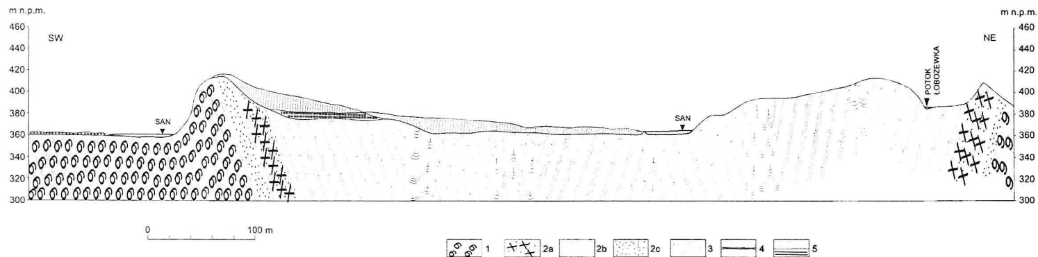
Rys. 2. Przekrój geologiczny przez synklinę Czulnia-Jawor (Dziewański 1973, z uzupełnieniami)
