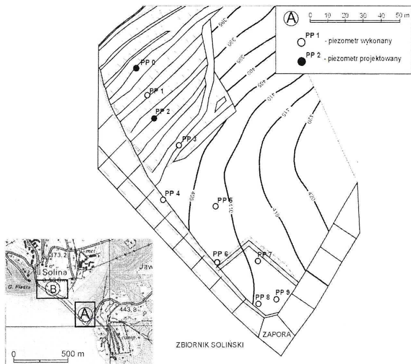
Rys. 7. Lokalizacja piezometrów wodowskazowych na prawym skrzydle zapory Solina (A) – marzec 2004 r. (wg dokumentacji technicznej ZEW, z uzupełnieniami)
