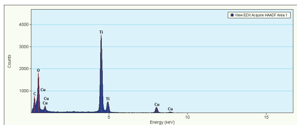
Fig. 5. EDS spectrum of TiO 2 nanopowder
