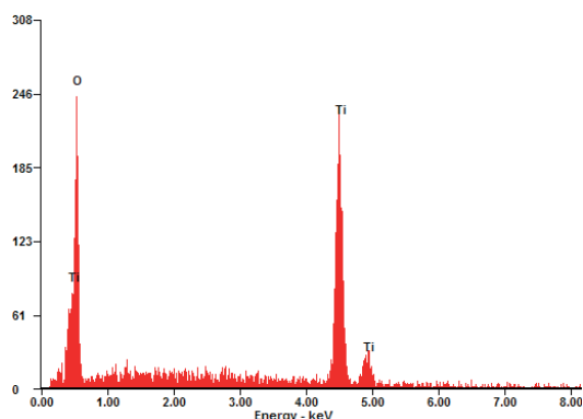
Fig. 7. EDS spectrum of TiO 2 micropowder
