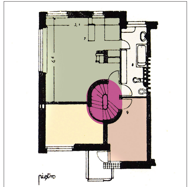
13. Dom własny na Żoliborzu w Warszawie, projekt B. i S. Brukalscy (realizacja 1928 r.), rzut parteru i pierwszego piętra. Źródło: „Architektura i Budownictwo”, 1931, s. 9 13. Barbara and Stanisław Brukalski, own home in Żoliborz, Warsaw (1928), the plan of the ground floor and the first floor. Source: “Architektura i Budownictwo”, 1931, p. 9
