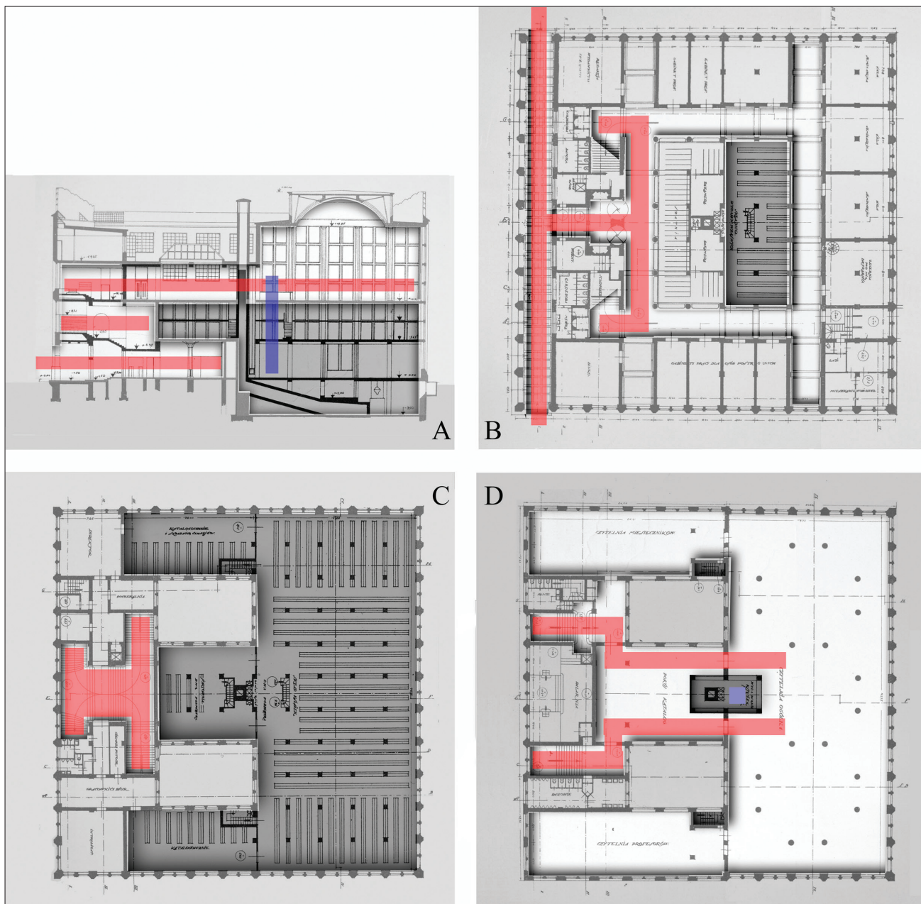
10. Biblioteka WSH, proj. J. Koszczyk-Witkiewicz (projekt 1924 r.), kolorami oznaczono: szary – magazyn książki, czerwony – droga czytelnika, niebieski – droga książki; A – przekrój; B – rzut parteru; C – rzut pierwszego piętra; D – rzut drugiego piętra. Źródło: „Architektura i Budownictwo”, 1933, s. 3–5
