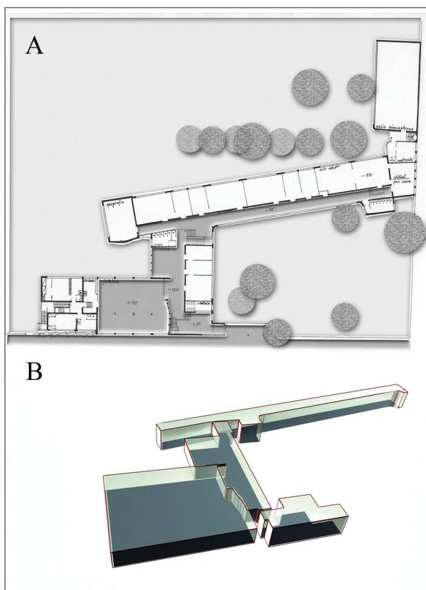
16. Gimnazjum im. E. Plater w Warszawie, projekt Romuald Gutt (1934 r.); A – rzut parteru; B – aksonometria przestrzeni wspólnej gimnazjum. Rys. autor 16. Romuald Gutt, E. Plater's Gymnasium, Warsaw (1934); A – ground floor plan; B – axonometric view of the gymnasium's common space. Author's drawing
