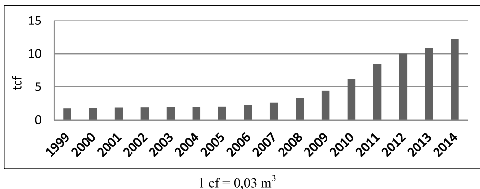
Rys. 1. Wydobycie węglowodorów niekonwencjonalnych w USA ( shale gas, tight gas ) w latach 1999–2014 (tcf = biliony stóp sześciennych)
