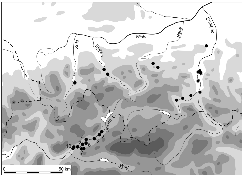
Fig. 3. Lusatian culture strongholds and upland settlements: 1 – Nižná; 2- Podbiel; 3 – Sedliacka Dubová; 4 – Oravský Podzámok; 5 – Mokrad; 6 – Medzibrodie; 7 – Vyšný Kubín – Ostrá skala; 8 – Vyšný Kubín-Tupá skala; 9 – Veličná; 10 – Istebné (after Čaplovič 1987; Gedl 1976)
