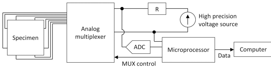
Fig. 4. Block diagram of the DAS.
