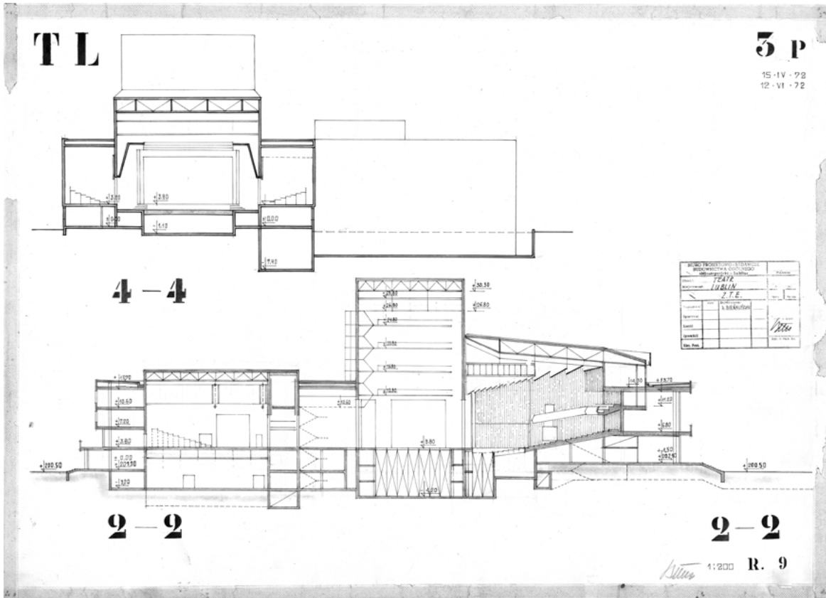
20. Przekrój podłużny Teatru Dramatycznego w Lublinie. Widoczne dwie sale teatralne, wielka i mała (eksperymentalna), 1972 (proj. S. Bieńkuński), Archiwum Urzędu Marszałkowskiego, fot. dzięki uprzejmości CSK
