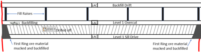
Fig. 8e. Backfilling Ring 1 void
