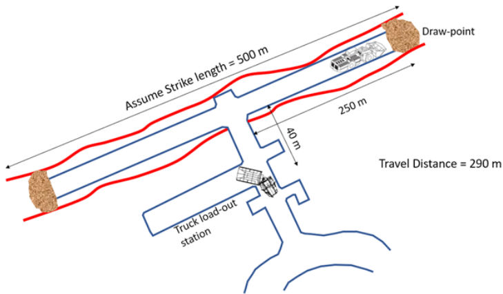
Fig. 13. LHD Cycle – Scenario 1
