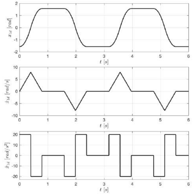
Fig.4. Desired trajectory
