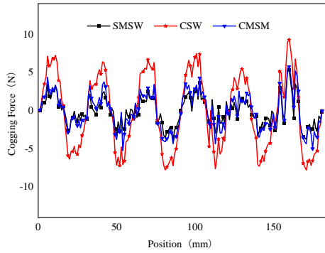
Fig. 15. Cogging force
