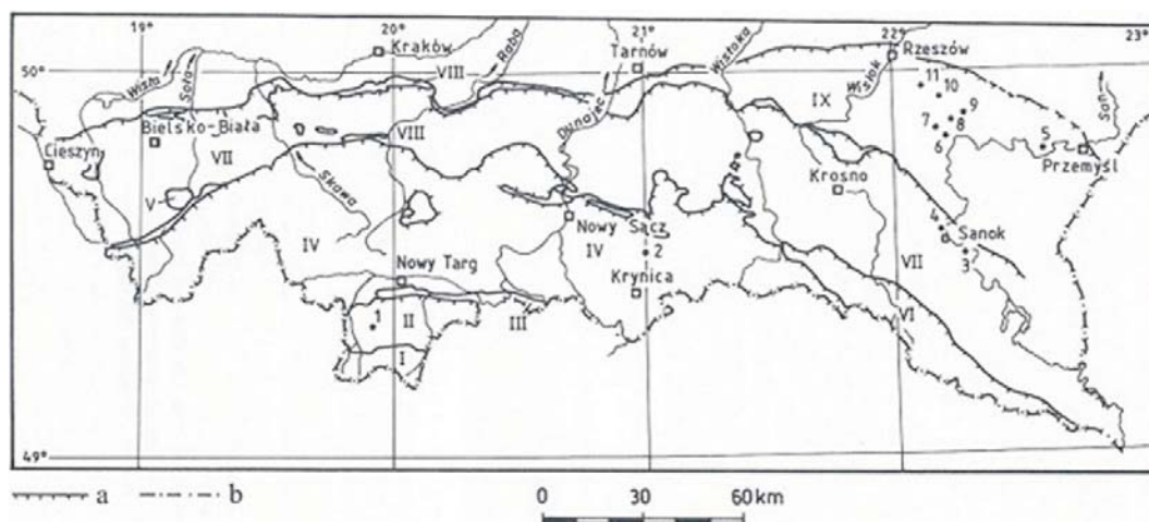
Rys. 1. Mapa rozmieszczenia bentonitów i skał pokrewnych w Karpatach fliszowych Polski
