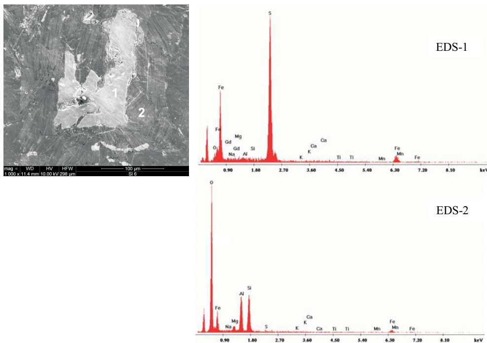
Rys. 6. Piryt (EDS-1) i schlorytzowany biotyt (EDS-2) w skale skaleniowo-kwarcowej ze złoża Strzeblów I
