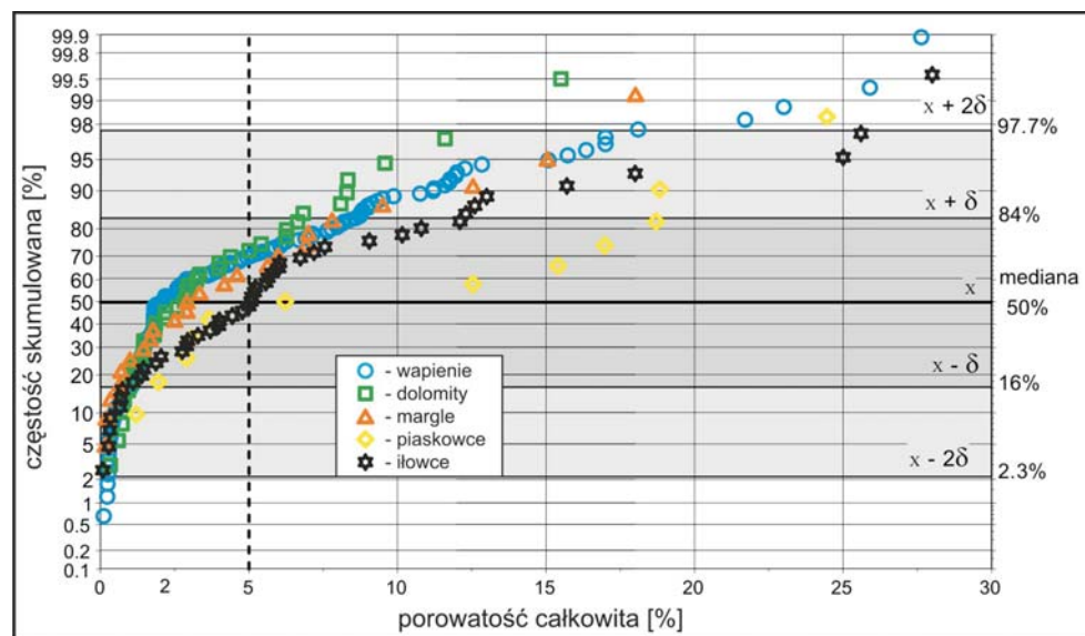
Rys. 3. Zmienność parametru porowatości całkowitej na wykresie prawdopodobieństwa w utworach wapienia muschelkalkowego dla poszczególnych typów litologicznych skał
