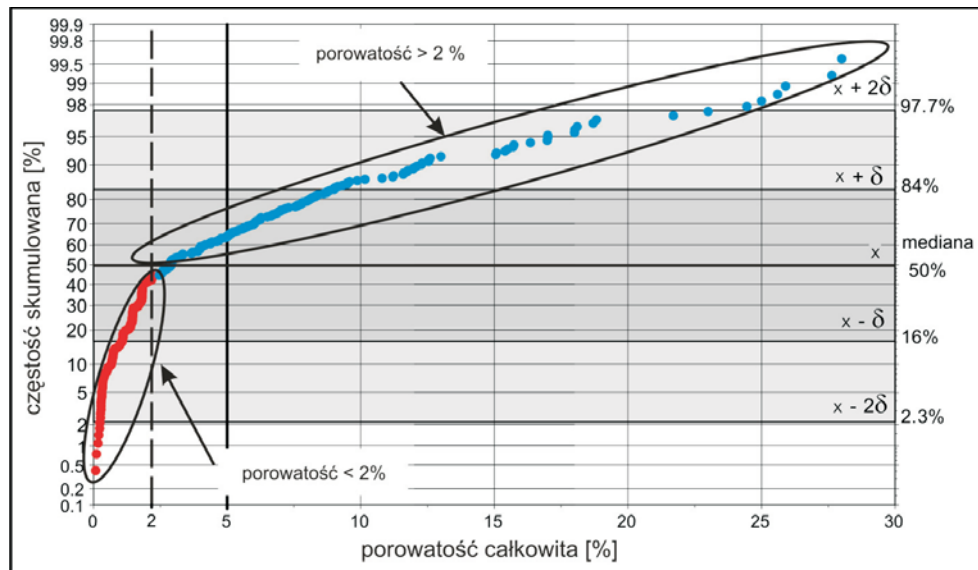
Rys. 2. Zmienność parametru porowatości całkowitej na wykresie prawdopodobieństwa w utworach wapienia muschelkalkowego
