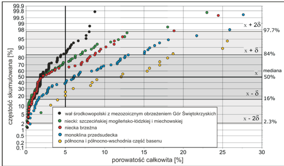
Rys. 9. Zmienność parametru porowatości całkowitej na wykresie prawdopodobieństwa w utworach wapienia muschelkowego w poszczególnych jednostkach strukturalnych Niżu Polskiego
