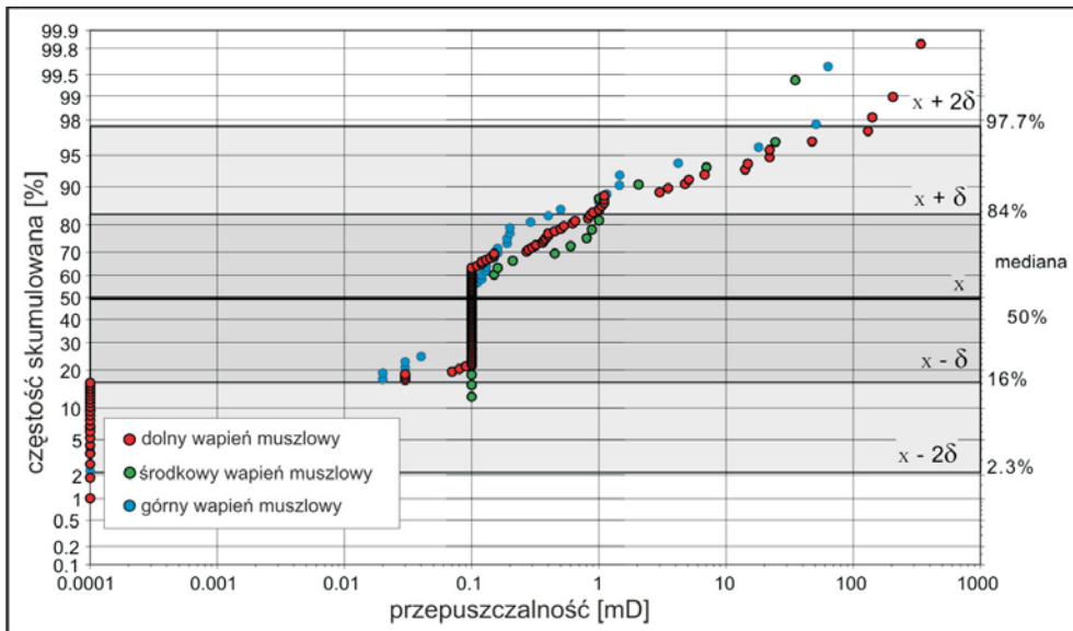
Rys. 12. Zmienność parametru przepuszczalności na wykresie prawdopodobieństwa w poszczególnych ogniwach wapienia muszlowego
