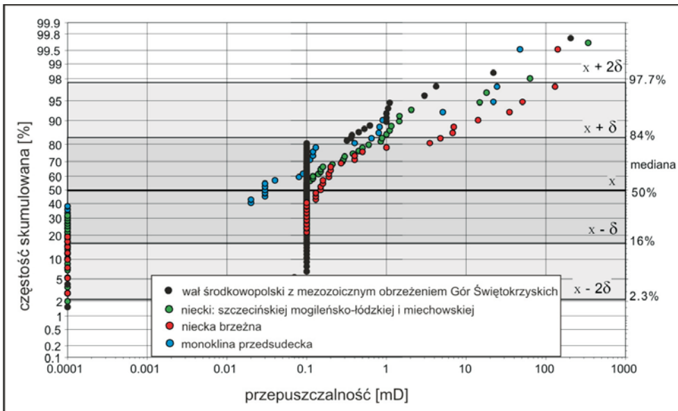
Rys. 10. Zmienność parametru przepuszczalności na wykresie prawdopodobieństwa w utworach wapienia muschelkowego w poszczególnych jednostkach strukturalnych Niżu Polskiego
