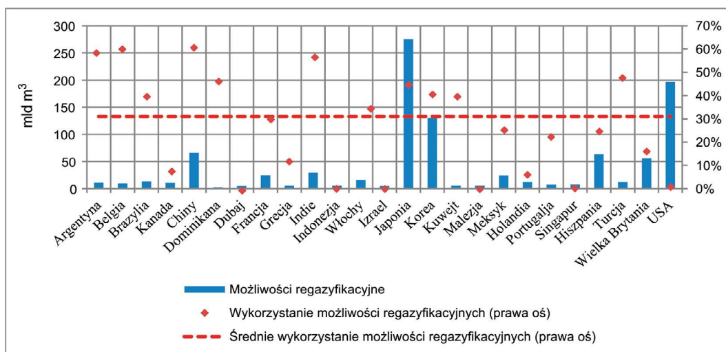
Rys. 4. Wykorzystanie możliwości regazyfikacyjnych przez wybrane państwa w 2013 r.
