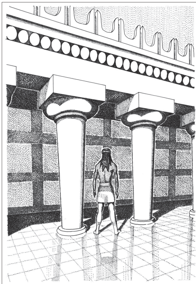
6. Porządek minojski – transformacja namiotowych podpór, symbol namiotu nieba. Rekonstrukcja wg własnej interpretacji 6. The Minoan order – a transformation of tent supports, a symbol of the tent of heaven. Reconstructed according to the Author's interpretation
