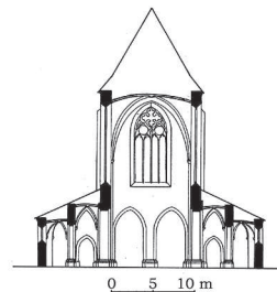
Lubiąż - kościół cysterski, prezbiterium 2 poł. XIII w., korpus 1 poł. XIV w.
