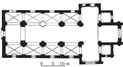
Rudy Raciborskie - kościół cysterski, 2 ćw. XIII w.
