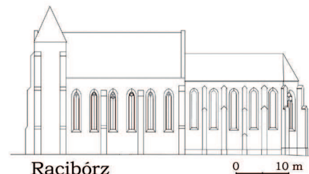
18. Widoki kościołów i rekonstrukcje elewacji podłużnych z XIII w. 18. Church views and reconstructions of longitudinal elevations from the 13 th c.
