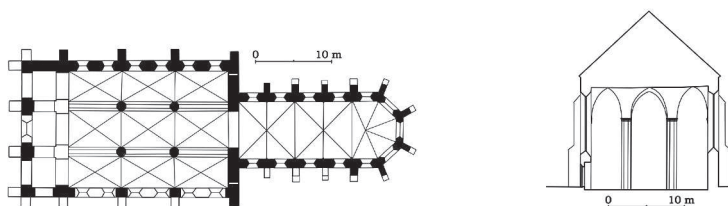
Racibórz - kościół parafialny p.w. NPM
