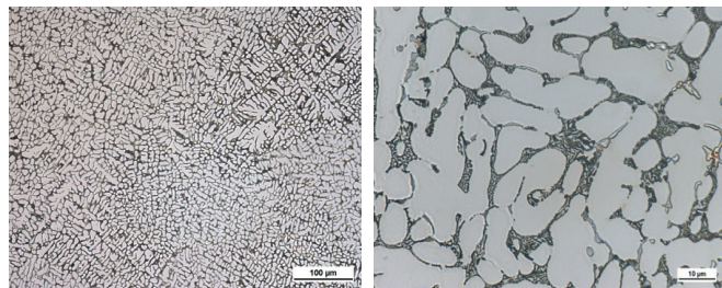
a) mag. 250× etch. 0.5 % HF b) mag. 1600× etch. 0.5 % HF
