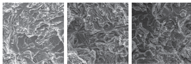
a) 0.0038 wt. % Sb b) 0.0094 wt. % Sb c) 0.0170 wt. % Sb
