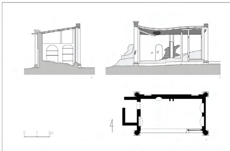
Ryc. 4. Witulin, oranżeria, a – przekrój, b – elewacja południowa, c – rzut, stan w roku 1983. Oprac. K. Boguszevska, (na podstawie: E. Mącik, Inwentaryzacja architektoniczno-konserwatorska , s. 636 c, WUOZ/Radzyń Podlaski, 1983).
